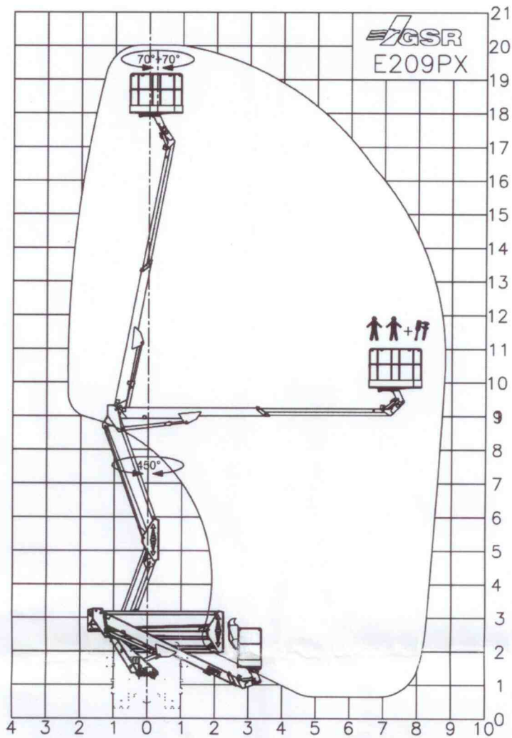
Pracovní diagram pracovnej plošiny GSR E209PX na podvozku Nissan Cabstar NT400.
